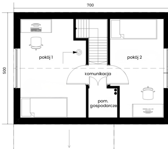
poddasze
