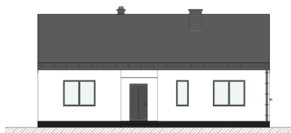
ELEWACJA 2
